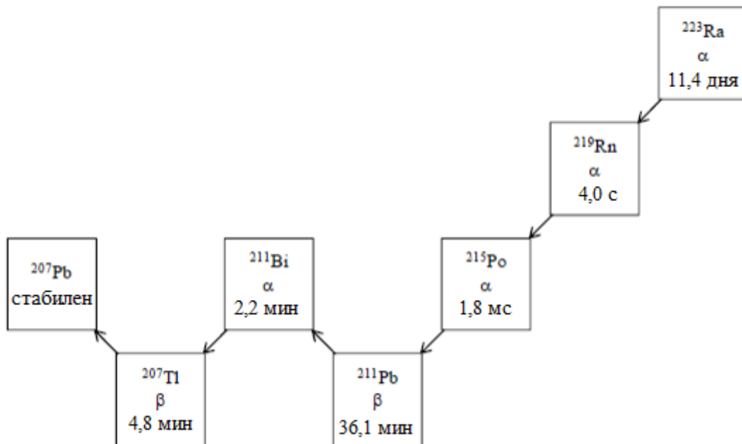
Рисунок 1. Цепочка радиоактивного распада радия-223 (с характером распада и параметрами периодов полураспада)
